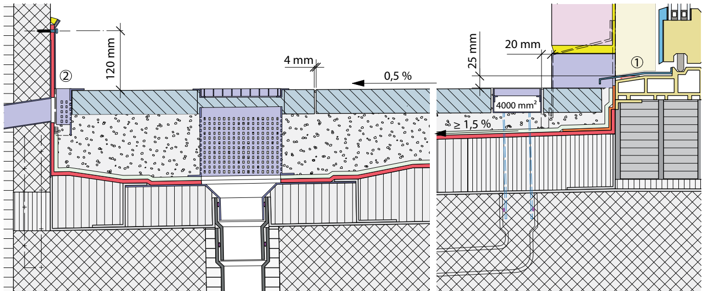
Abb. 14: Ausnahmeregelung Gefälle Plattenbelag < 1,5 %;
