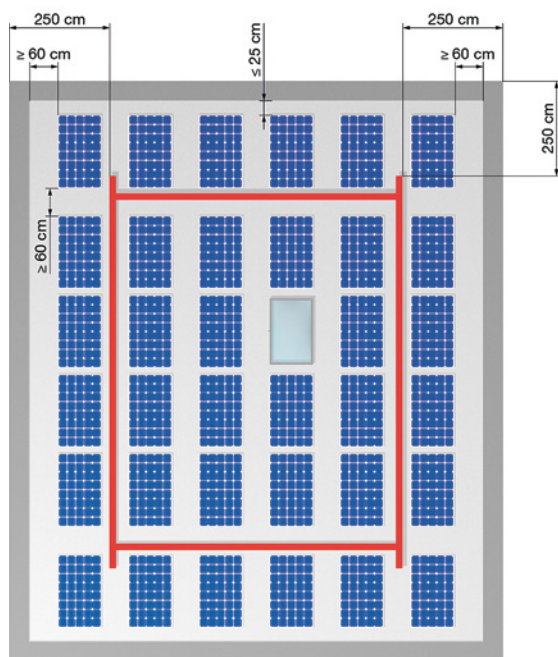
Bild 7 Beispiel «Omega-Form»
