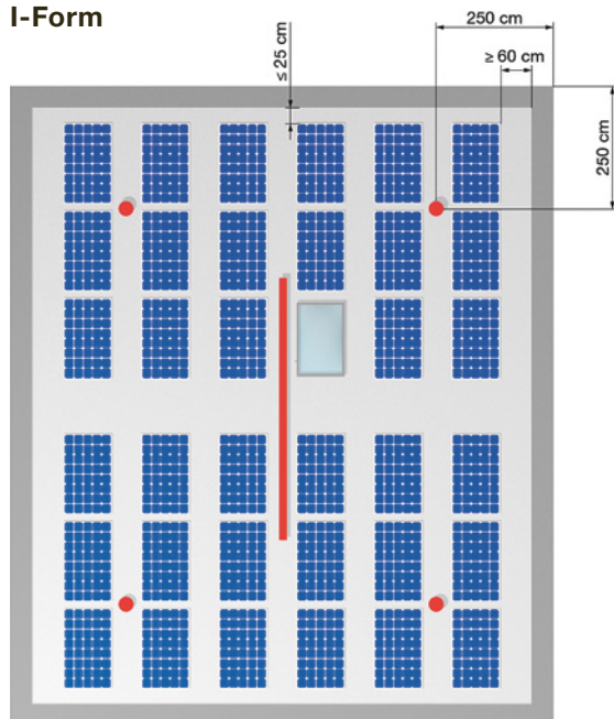
Bild 9 Beispiel «I-Form»
