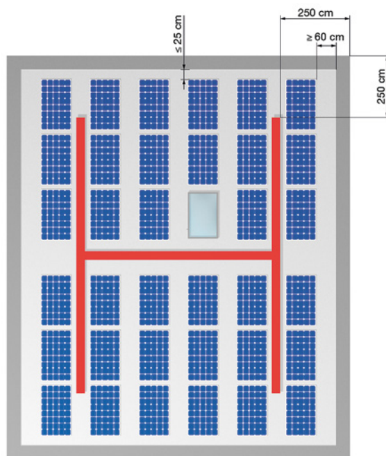
Bild 8 Beispiel «H-Form»
