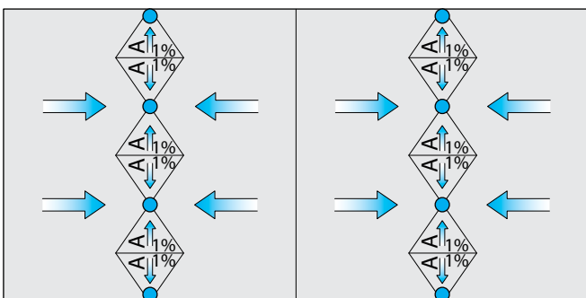
Abb. 11: Jeweils ein zweiseitiges Gefälle von 1,5% zu den Dachwassereinläufen, z.B. bei Metall- oder Holzunterkonstruktionen, mit einer aufgesetzten Gefällezugung (A) zwischen den Einläufen. Dachwassereinläufe an die sanitären Entwässerungsleitungen angeschlossen.
