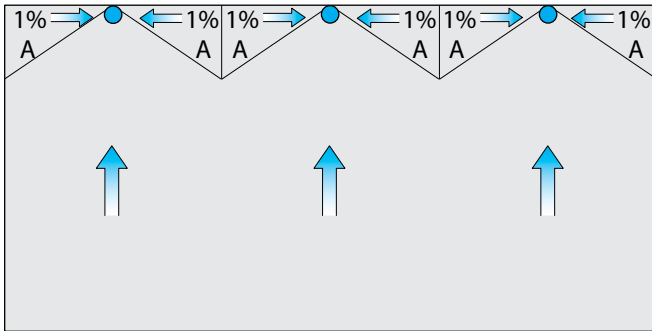
Abb.9: Einseitiges Gefälle von 1,5% z.B. zur Brüstung, zwischen den Einläufen eine aufgesetzte Gefällezugung (A). Dachwassereinläufe z.B. durch Speier und Ablaufrohre an der Fassade nach unten geführt.
