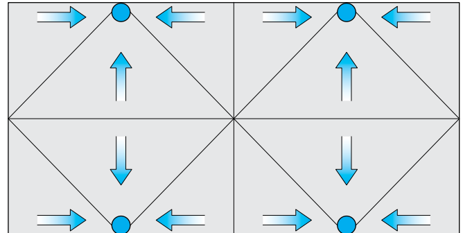
Abb. 6: Allseitig gleichmässiges Gefälle von 1,5 %, Dachwassereinflüsse, z. B. durch Speier und Ablaufrohre an der Fassade nach unten geführt.
