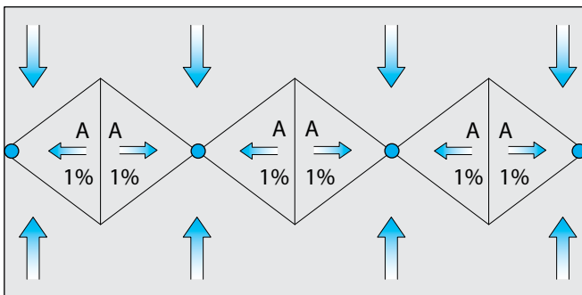
Abb. 10: Zweiseitiges Gefälle von 1,5% in die Mitte, zwischen den Einläufen eine aufgesetzte Gefälledämmung (A), Dachwassereinläufe an die sanitären Entwässerungsleitungen angeschlossen.
